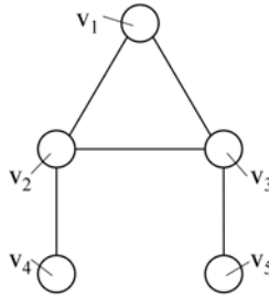
Рис. 2: Пример графа.
