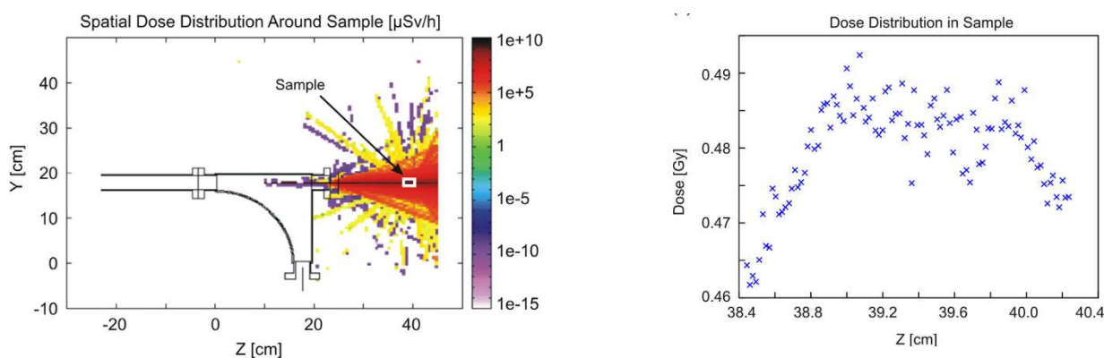
Рис. 23. Расчетное пространственное распределение поглощенной дозы на экспериментальной точке H1 и поглощенной дозы в биологическом образце вдоль продольной оси, указывающей направление пучка (справа).
