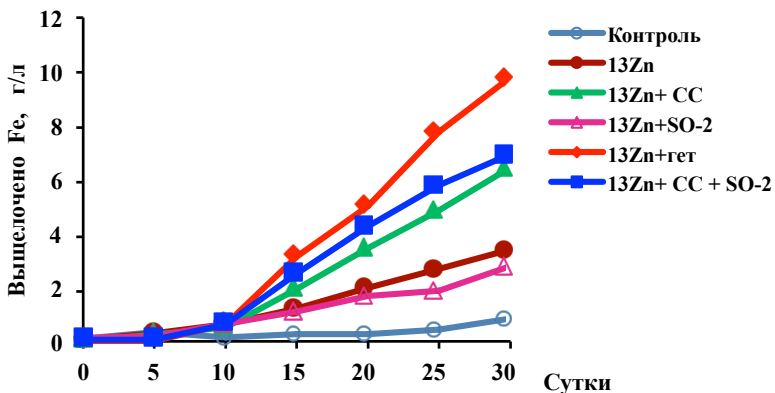
Рис. 4. Окисление пирита чистой культурой Acidithiobacillus sp. 13Zn и ассоциациями с железоокисляющей и сероокисляющей бактериями L.ferriphilum CC и At.albertensis SO-2 ( FeS_2 - 4%, pH 1.8, t - 30°C)
