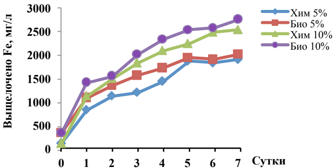
Рис. 7. Экстракции железа при химическом выщелачивании пирита (pH 1.8, t = 40°C)
