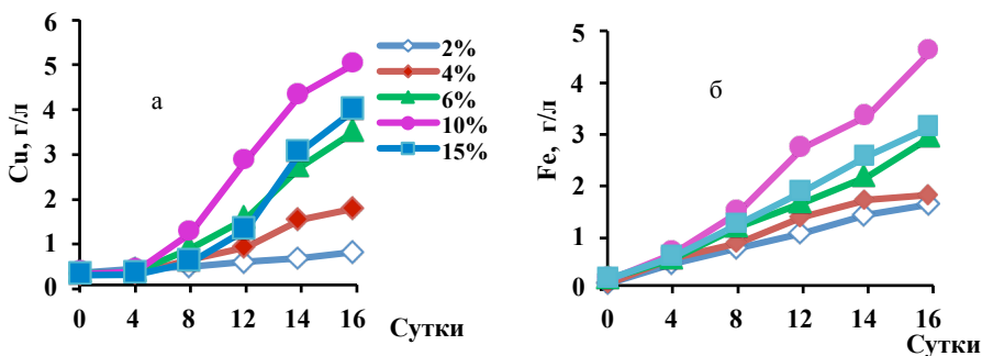
Рис. 2. Влияние концентрации халькопирита на выщелачивание меди (а) и железа (б) Acidithiobacillus sp. 13Zn (рН 1.7, t - 35°C)
