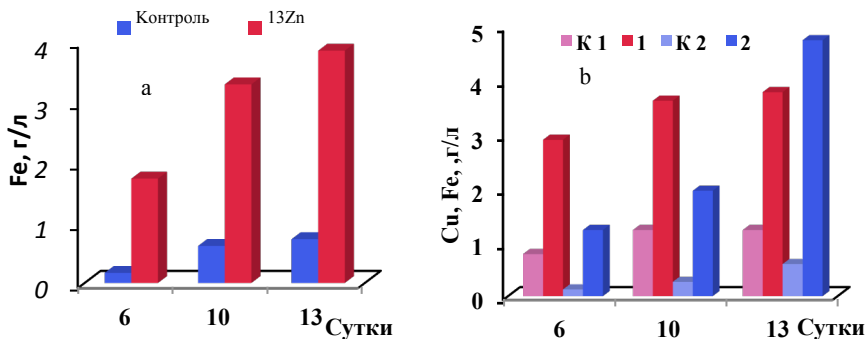
Рис. 1. Выщелачивание Дрмбонской руды (а) и медного концентрата (б) Acidithiobacillus sp. 13Zn (ПП 10%, рН 2.0, t-37°C); K1, K2 - контроль без бактерий
